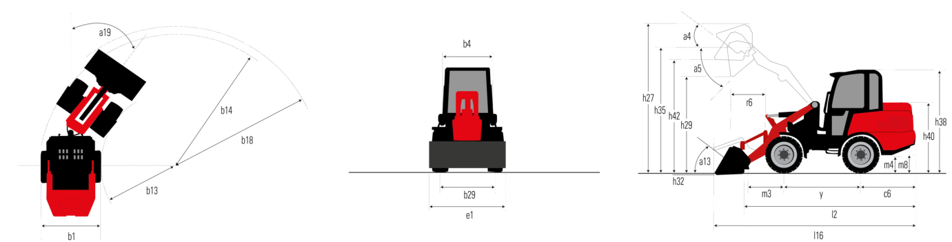
MLA 3-25 H-C - Tekening met afmetingen
