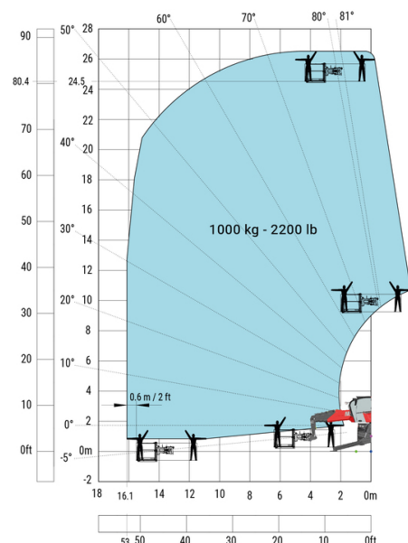
Rotatie op verlaagde stabilisatoren met 1000 kg platform
