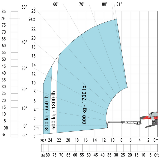
Rotatie op verlaagde stabilisatoren met 365 kg platform
